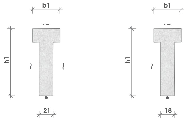
Поглед 1-1
