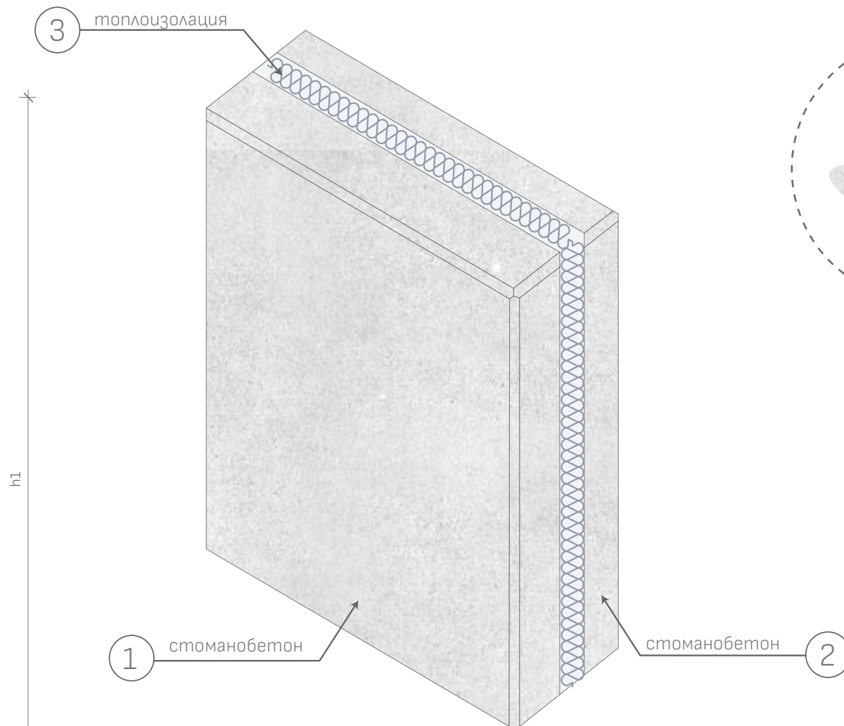
Детайл "А"
